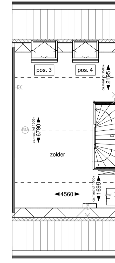
Tweede verdieping
