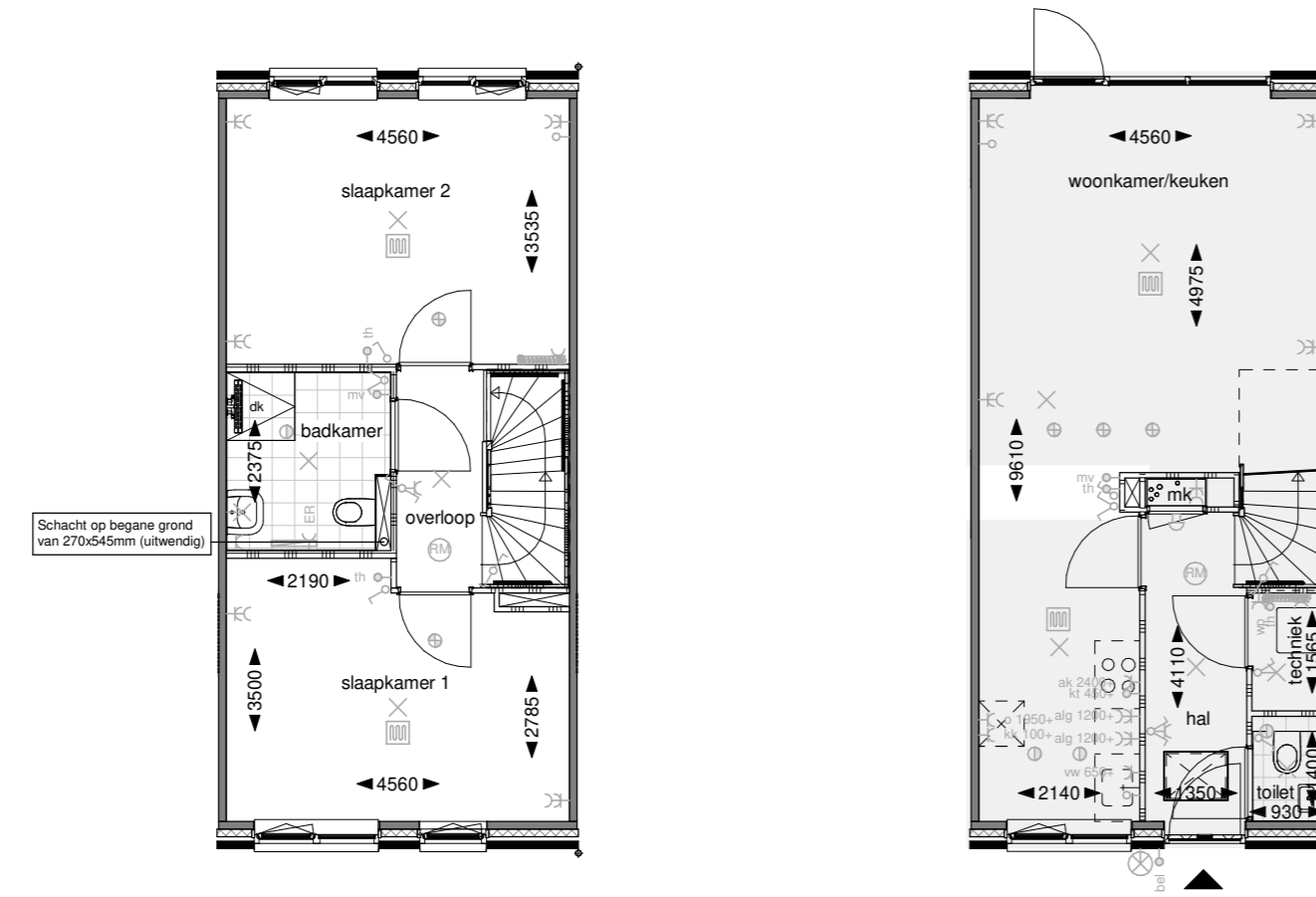
Eerste verdieping
