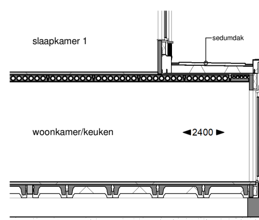
Doorsnede
