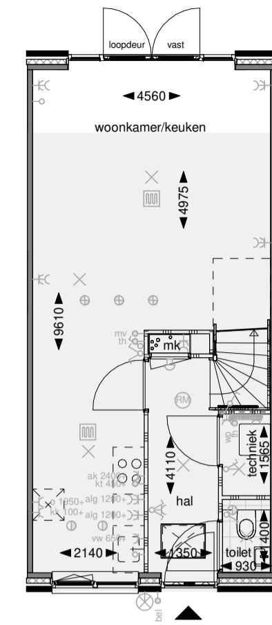
Begane grond
