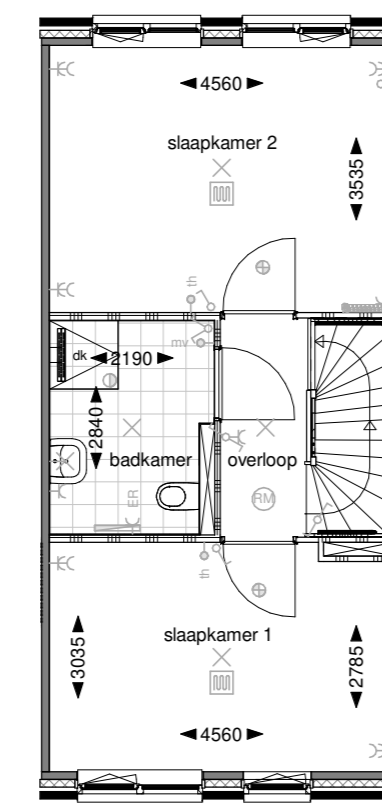
Eerste verdieping
