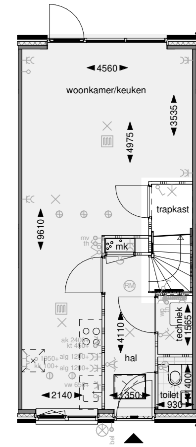
Begane grond
