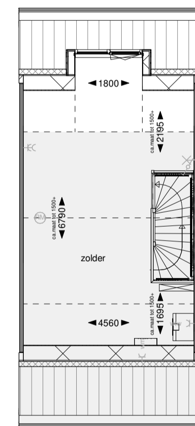
Tweede verdieping
