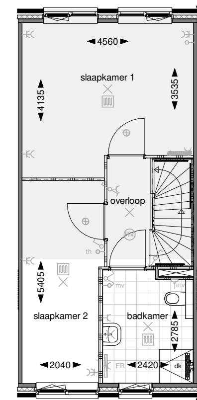
Eerste verdieping
