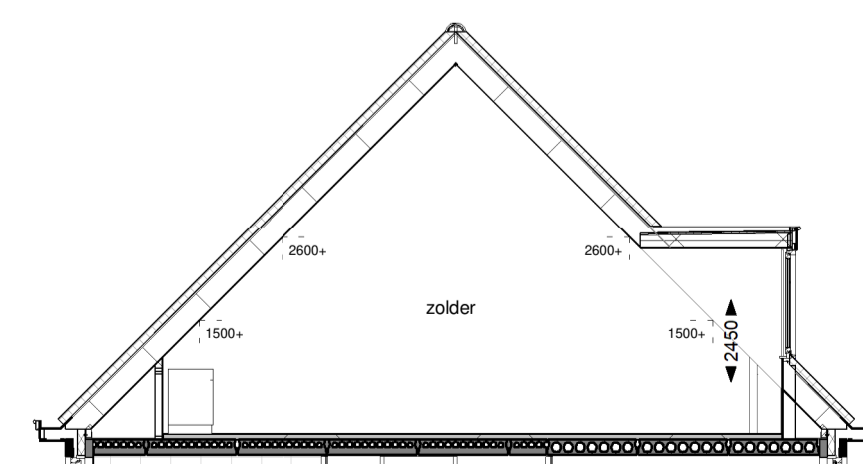
Doorsnede
