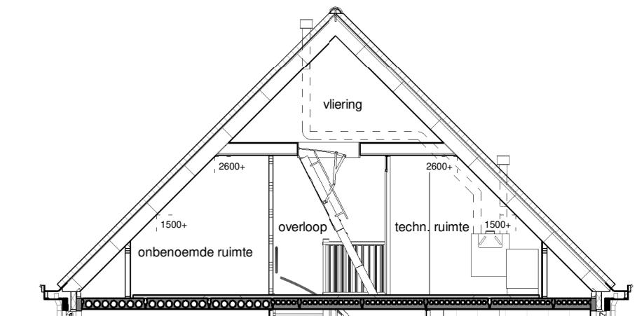
Doorsnede
