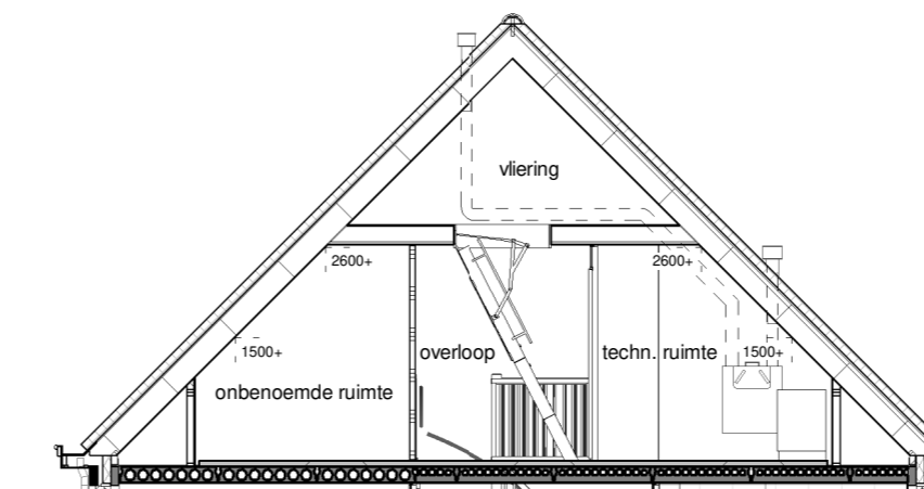
Doorsnede
