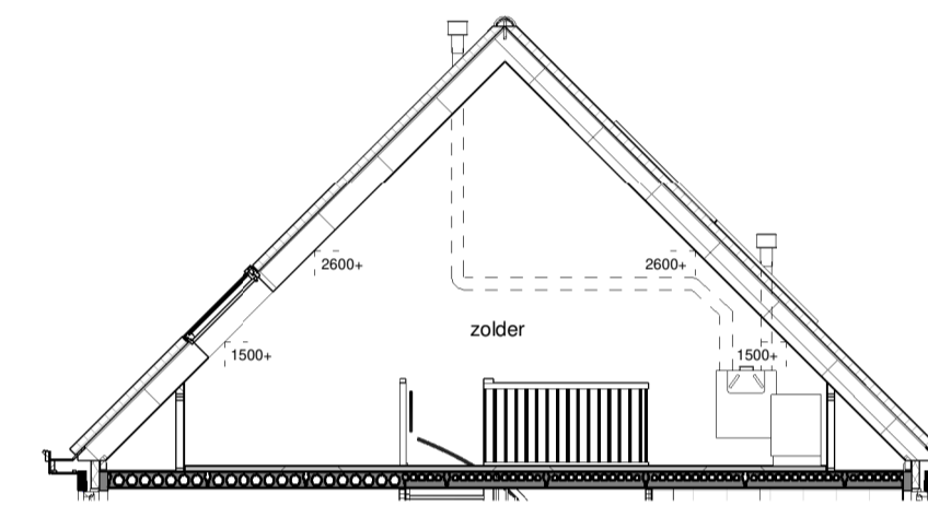
Doorsnede
