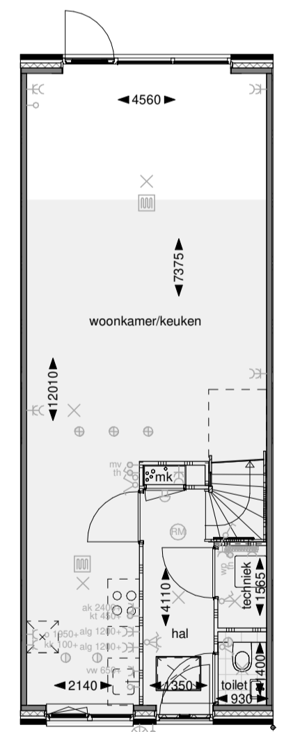
Begane grond
