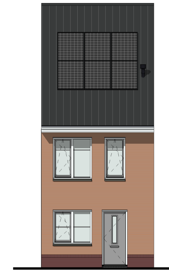
Voorgevel
