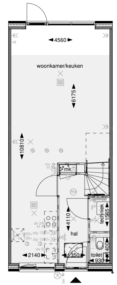
Begane grond
