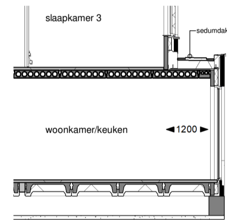
Doorsnede
