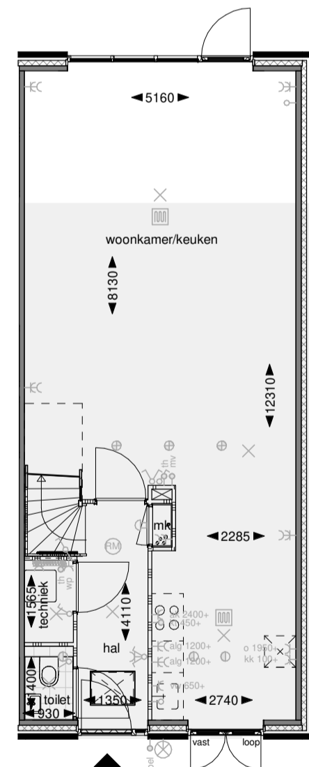
Begane grond
