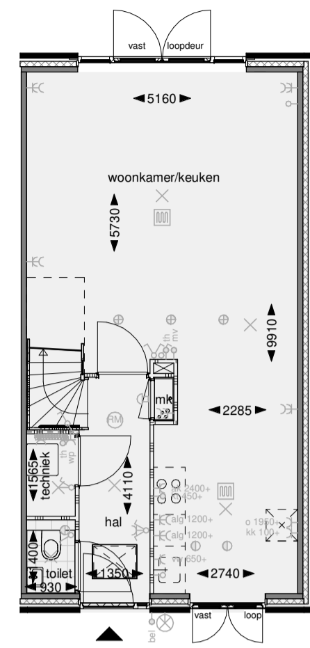
Begane grond
