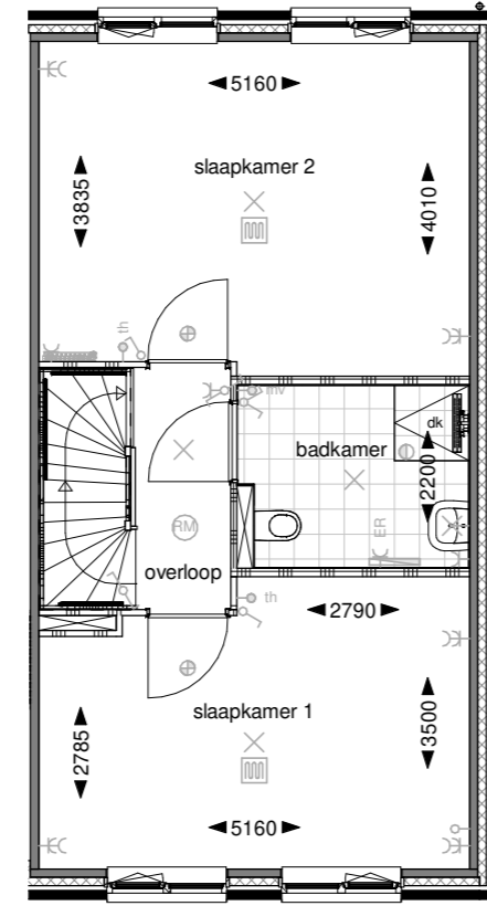
Eerste verdieping
