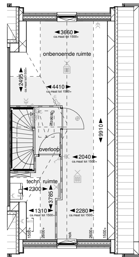
Tweede verdieping
