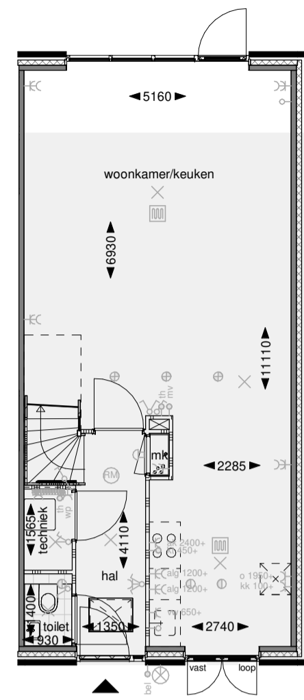
Begane grond
