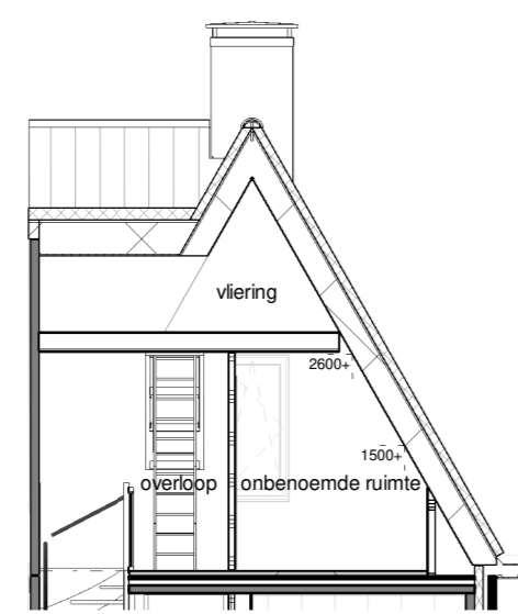
Doorsnede
