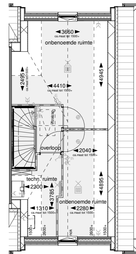
Tweede verdieping
