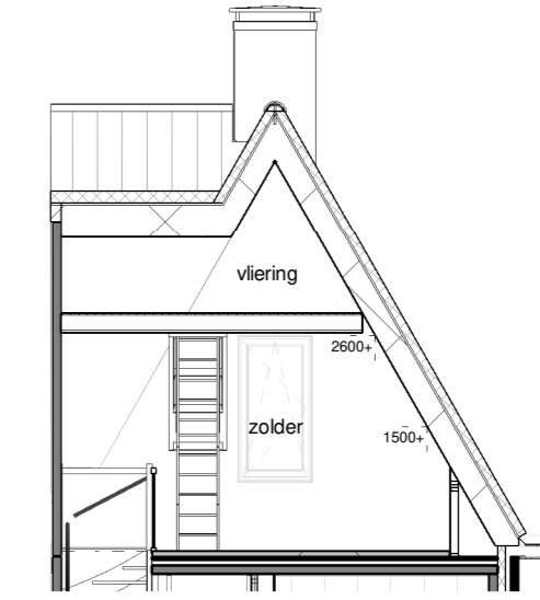
Doorsnede
