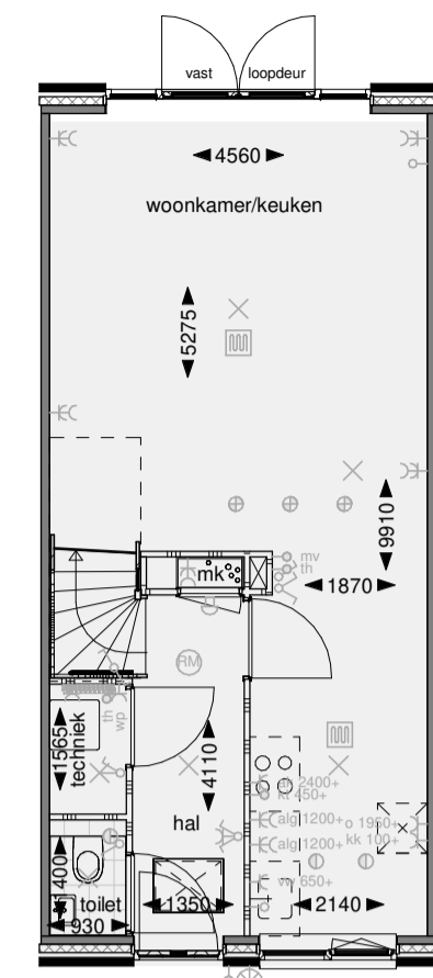
Begane grond
