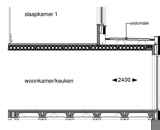
Doorsnede
