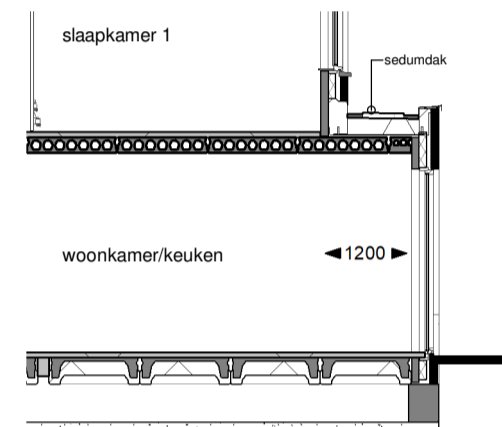
Doorsnede
