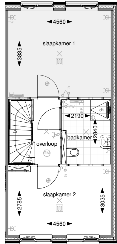
Eerste verdieping
