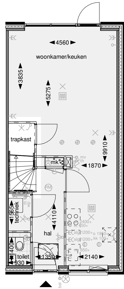
Begane grond
