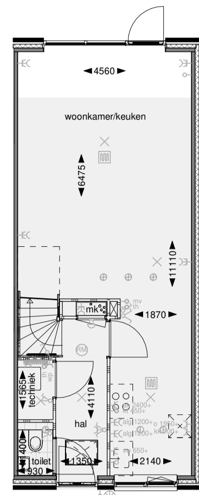
Begane grond
