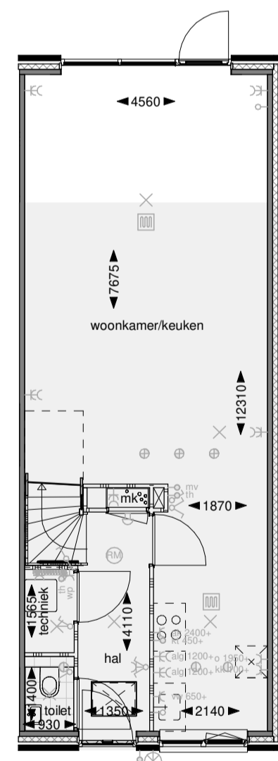
Begane grond
