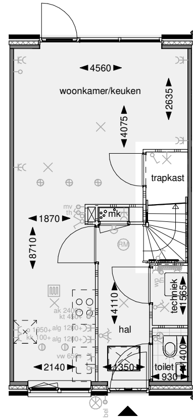
Begane grond
