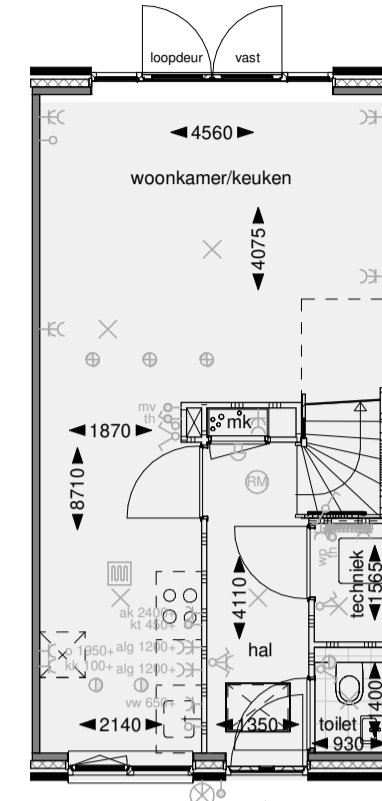
Begane grond
