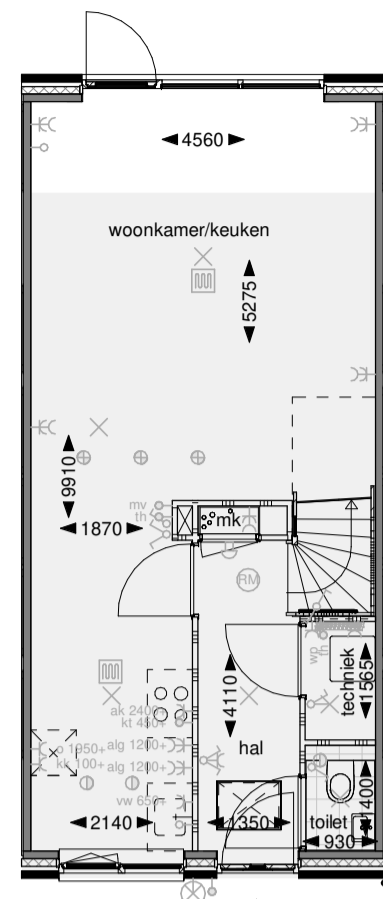
Begane grond
