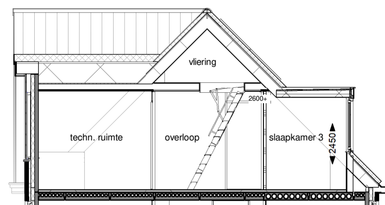
Doorsnede
