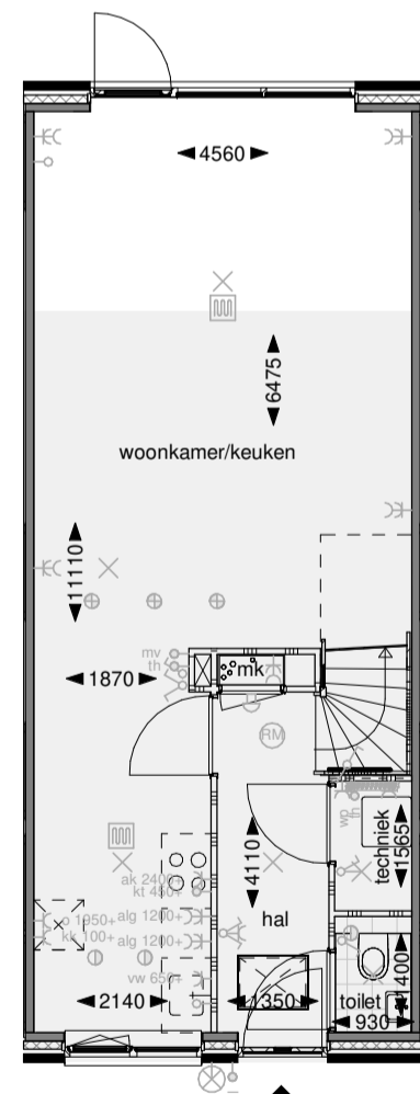
Begane grond
