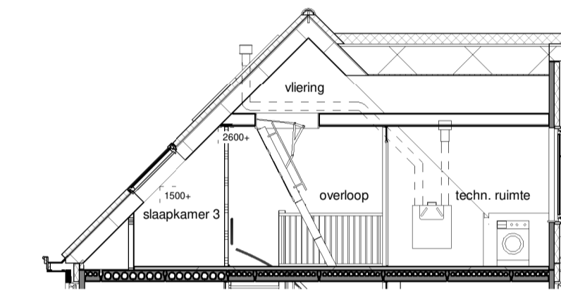
Doorsnede
