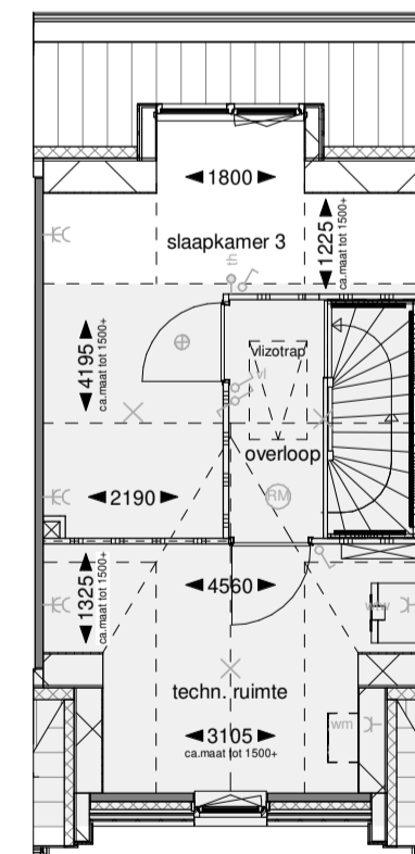
Tweede verdieping
