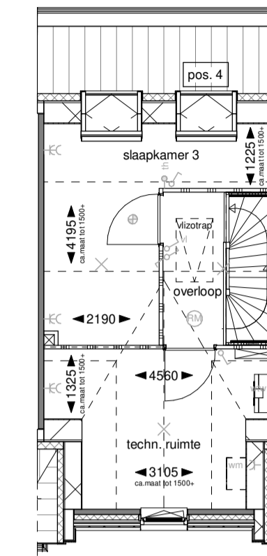
Tweede verdieping
