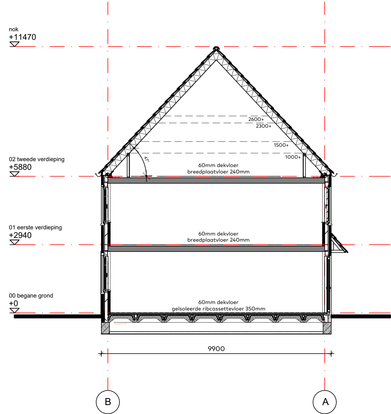
Doorsnede
