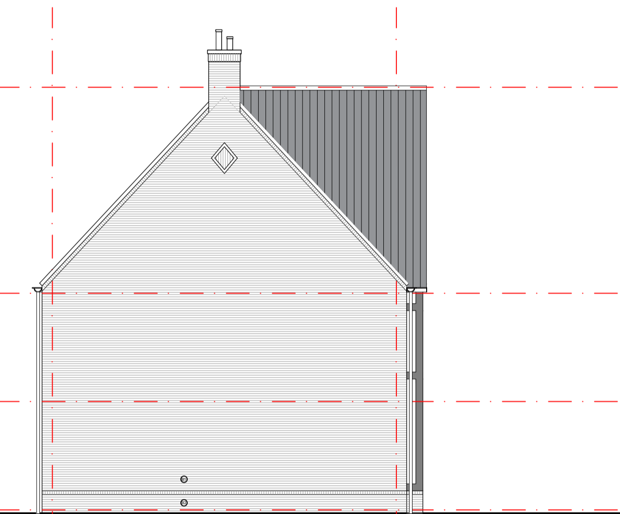
Zijgevel rechts, blok D
