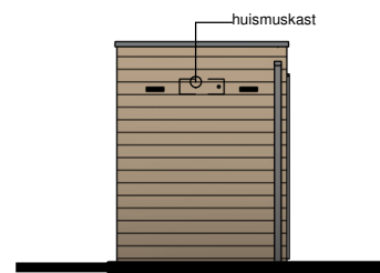
Poortanzicht
