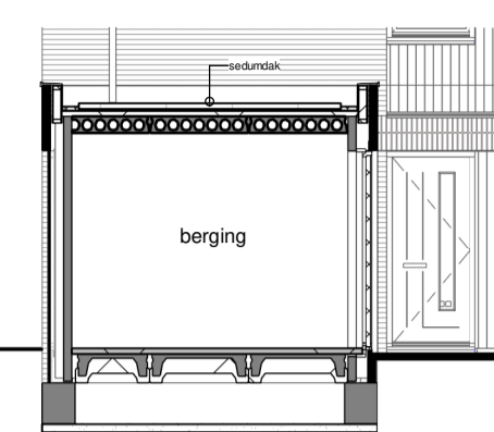
Fragment doorsnede
