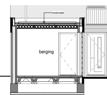
Fragment doorsnede
