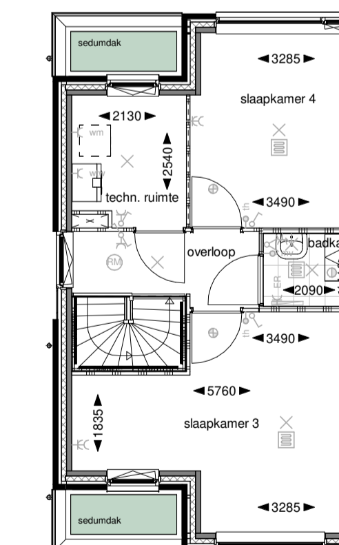
Tweede verdieping
