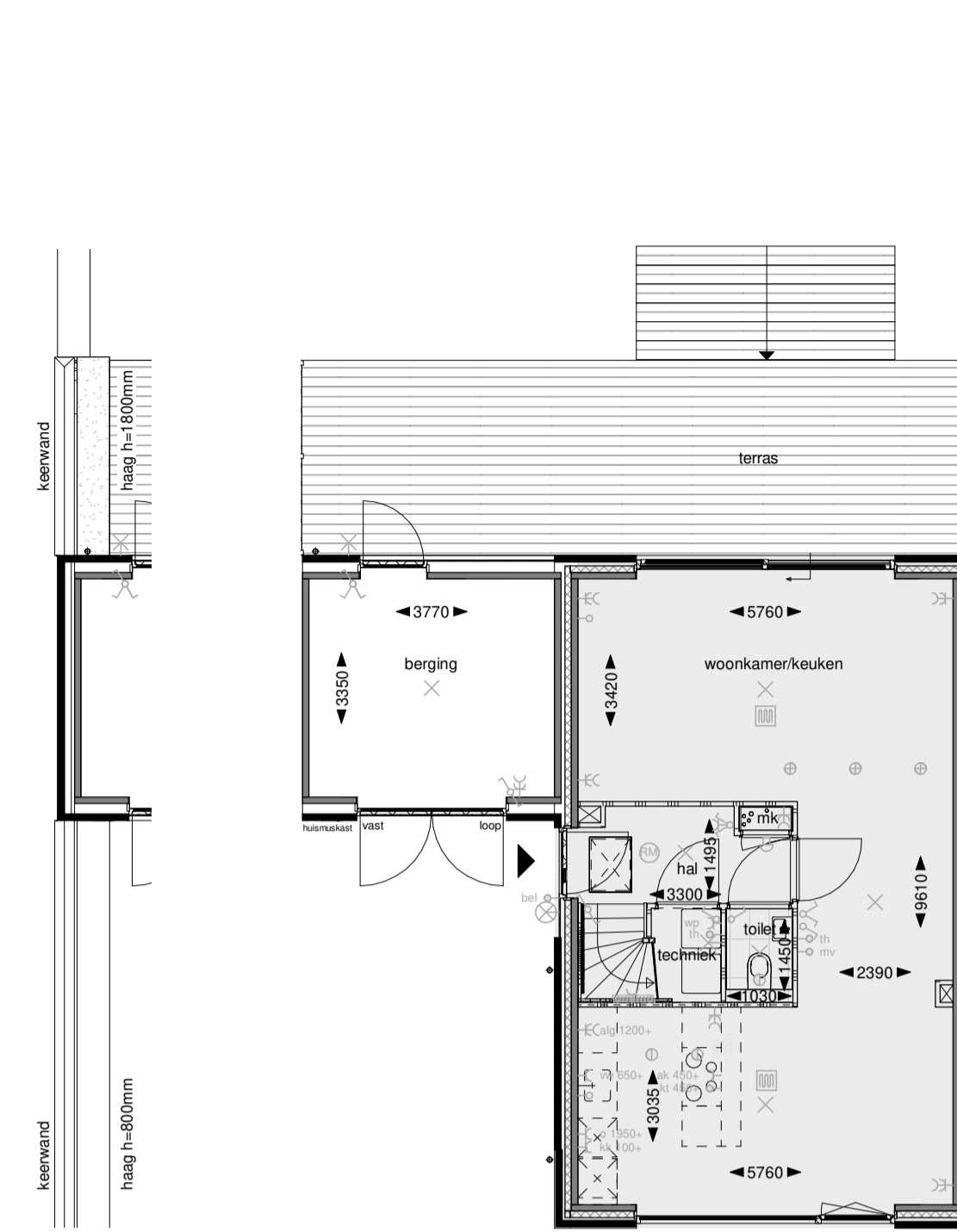
Begane grond Fragment kopgevel eindwoningen
