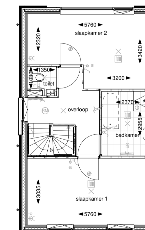
Eerste verdieping
