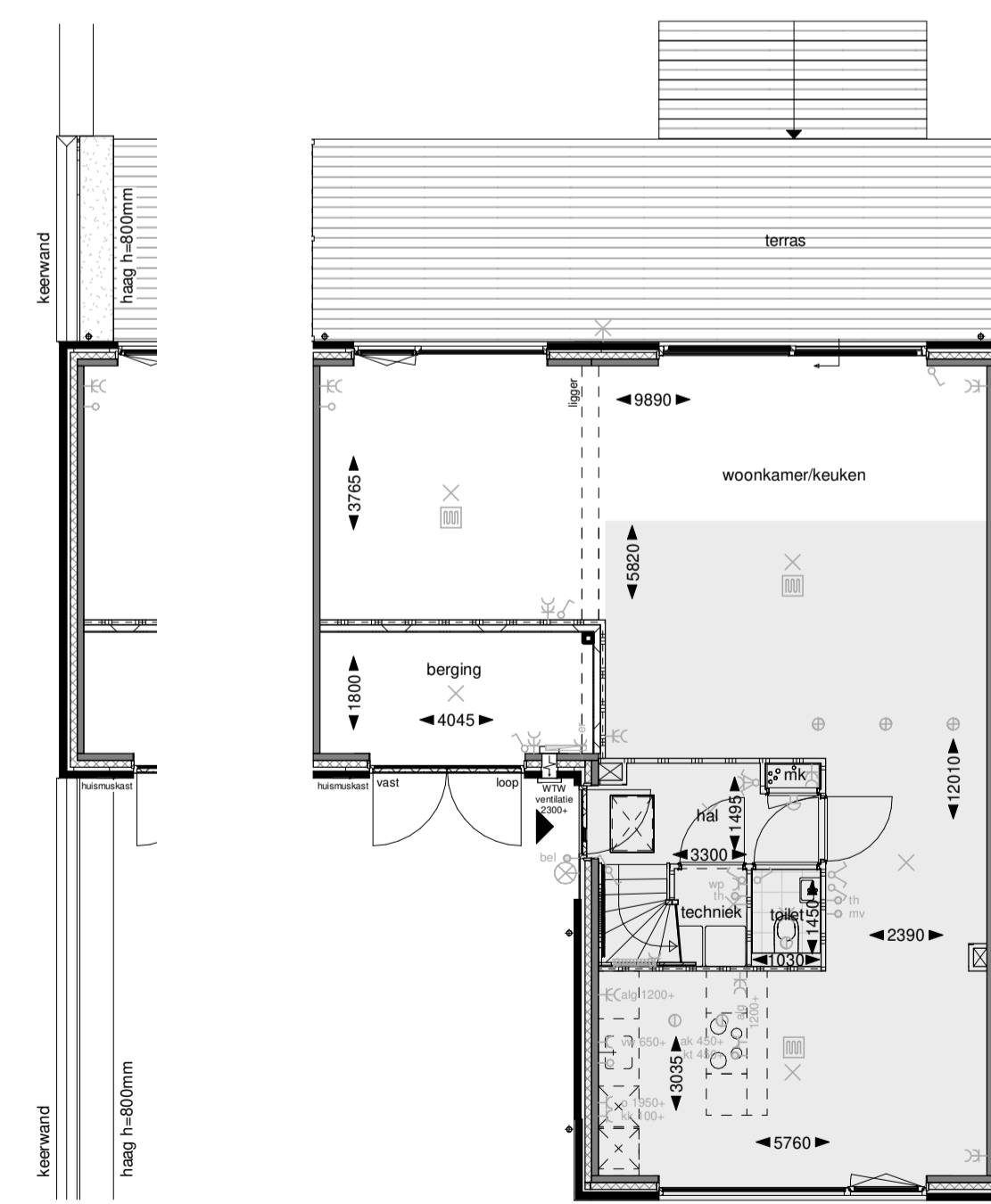
Begane grond Fragment kopgevel eindwoningen
