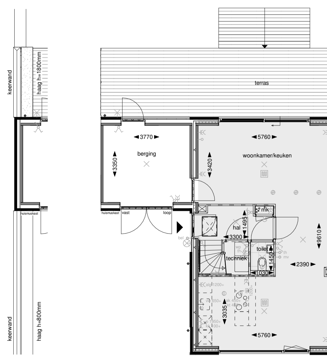
Begane grond
