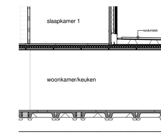
Fragment doorsnede
