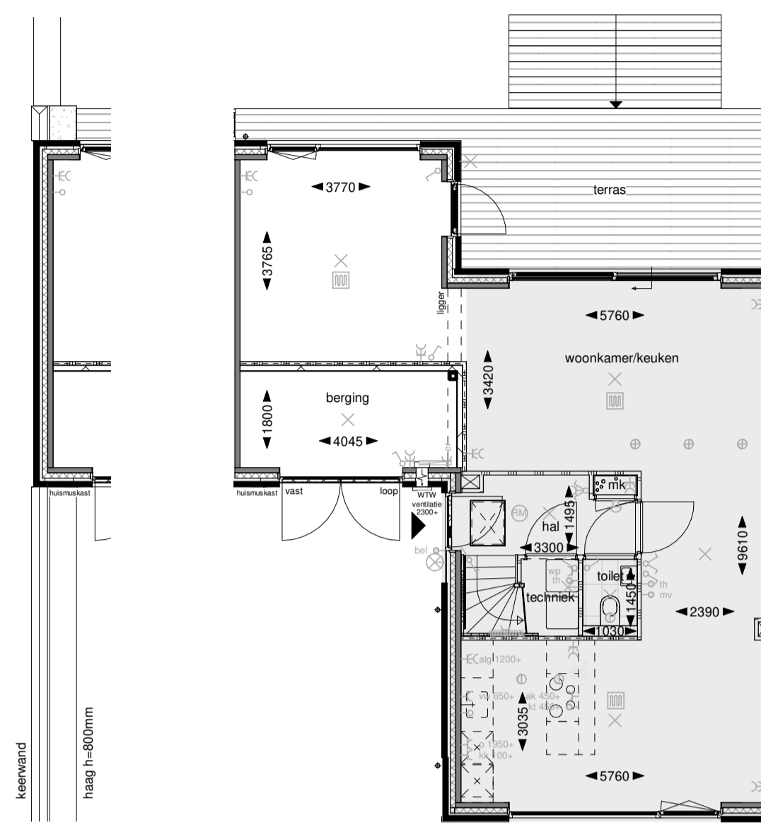
Begane grond
