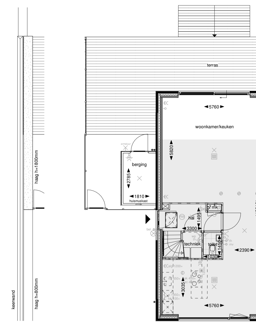
Begane grond Fragment kopgevel eindwoningen
