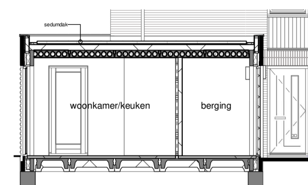
Fragment doorsnede
