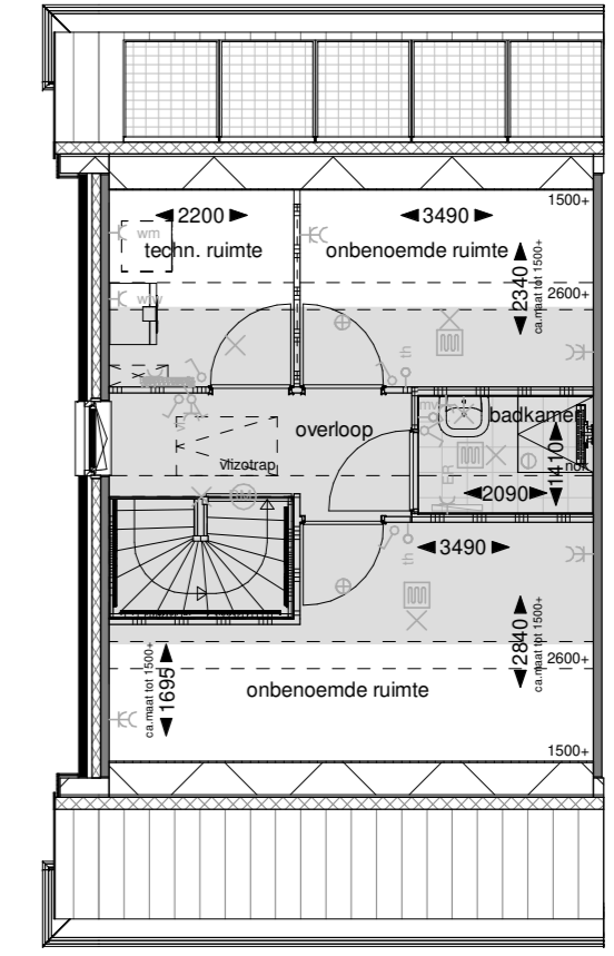
Tweede verdieping
