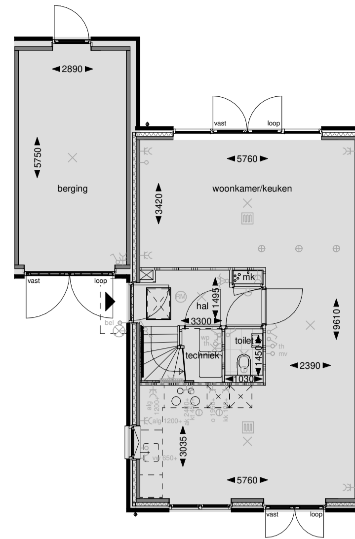
Begane grond
