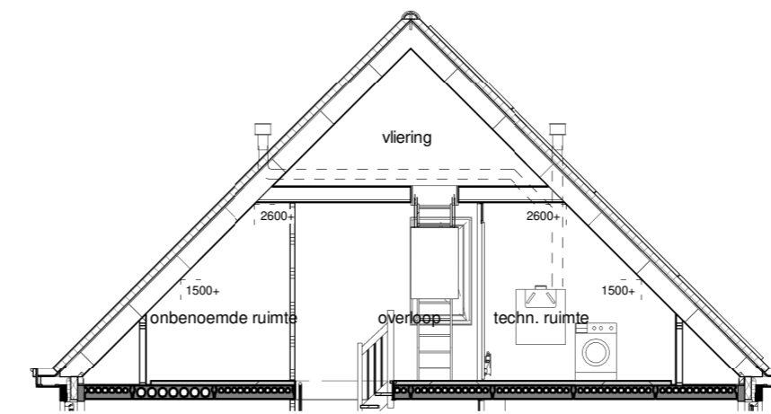
Doorsnede
