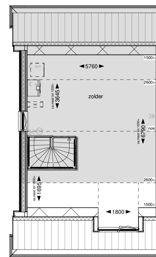
Tweede verdieping
