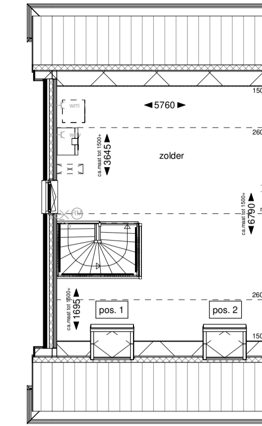
Tweede verdieping
