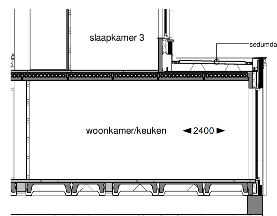
Doorsnede
