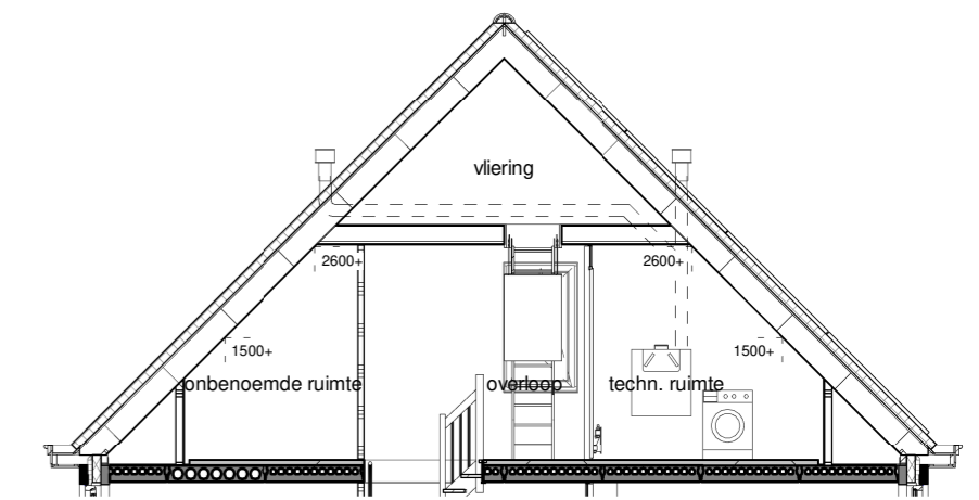
Doorsnede
