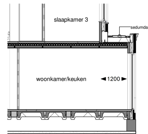
Doorsnede
