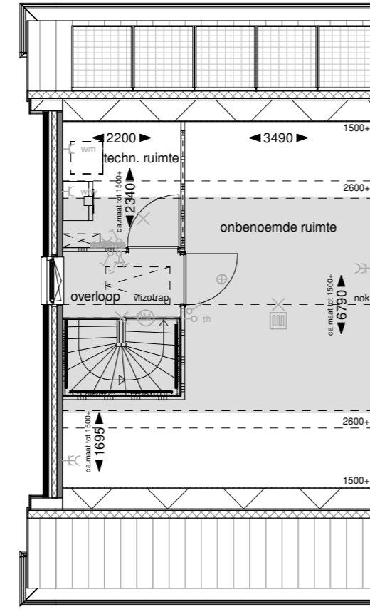
Tweede verdieping
