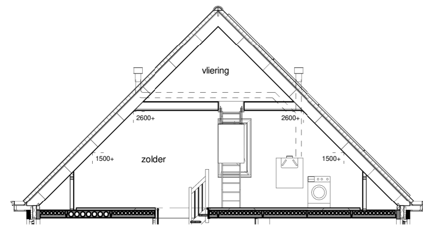
Doorsnede
