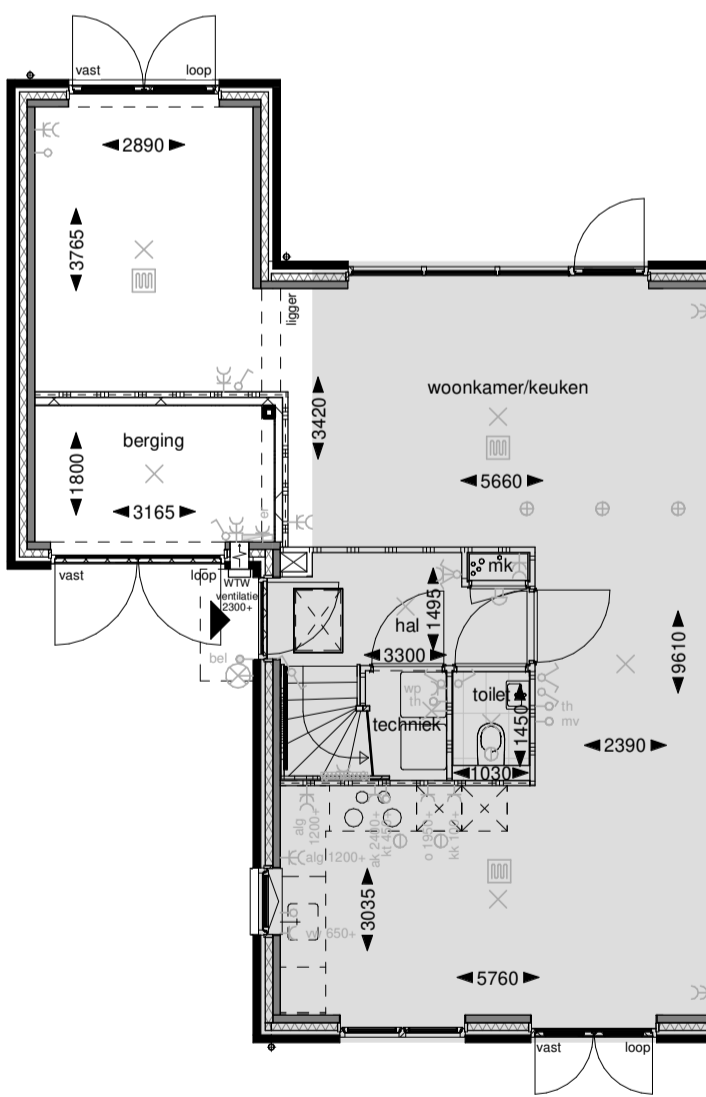
Begane grond
