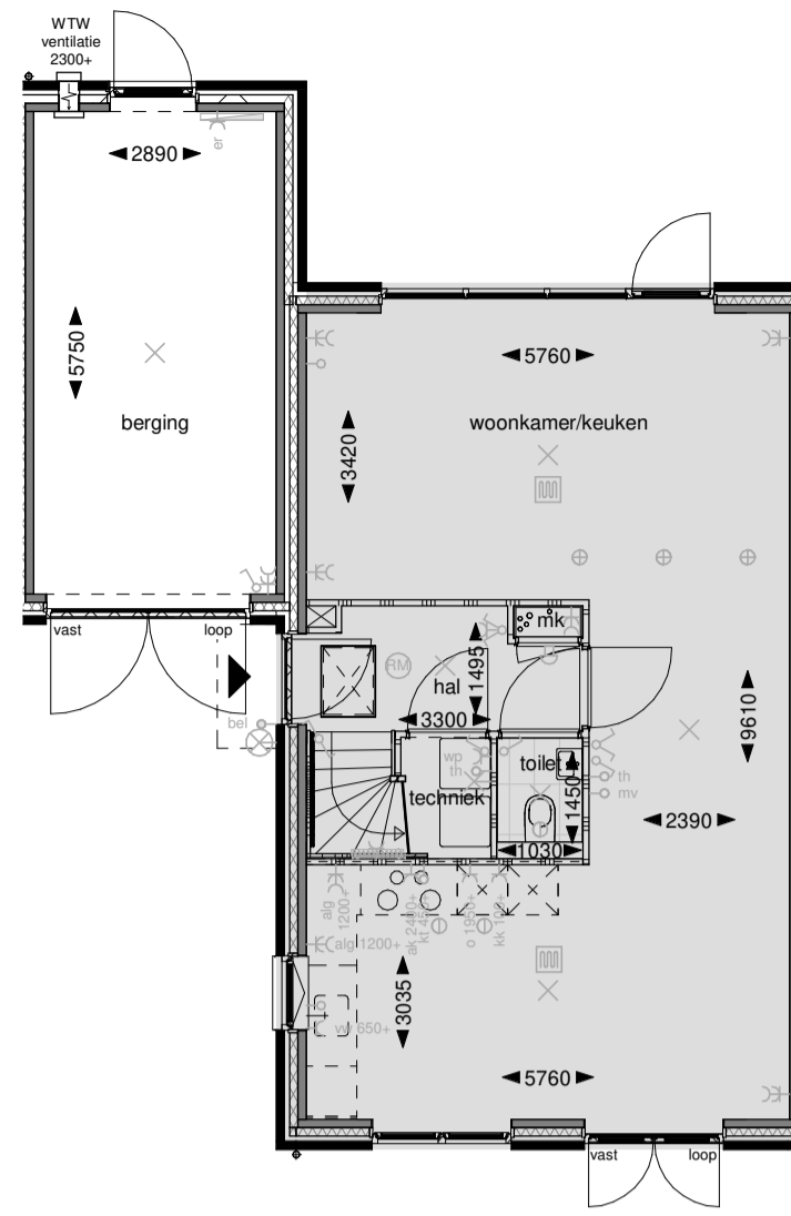
Begane grond
