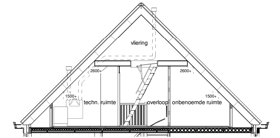
Doorsnede
