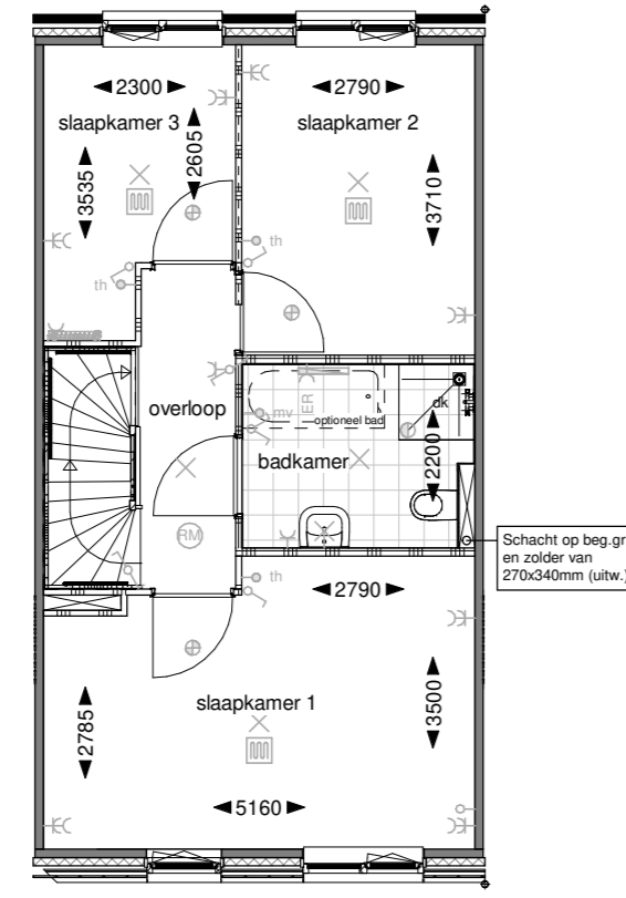
Eerste verdieping
