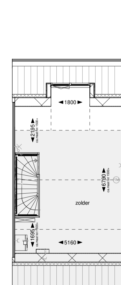
Tweede verdieping
