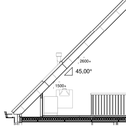
Doorsnede
