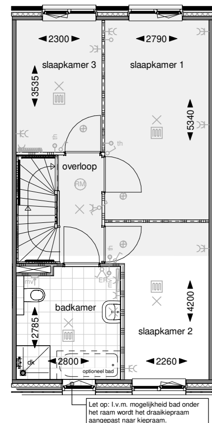
Eerste verdieping
