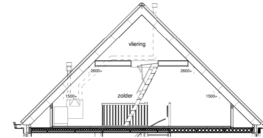
Doorsnede
