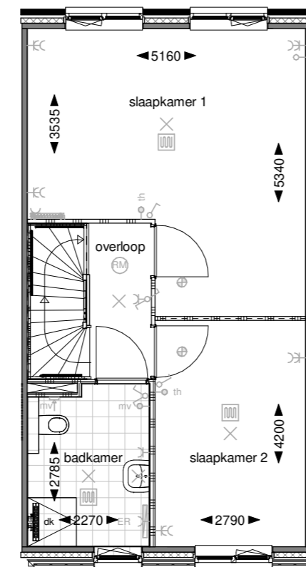
Eerste verdieping
