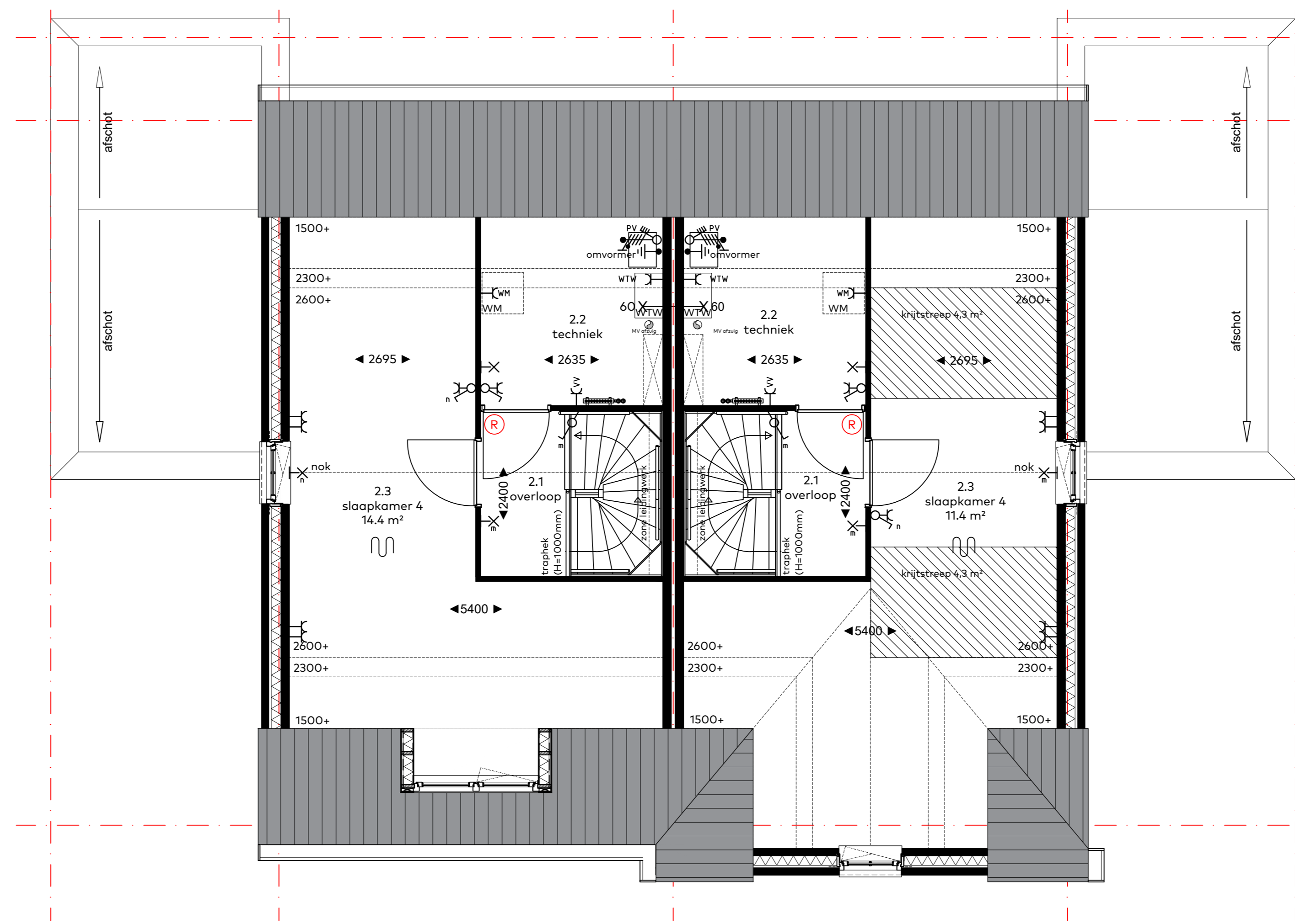
Tweede verdieping, blok E en F
