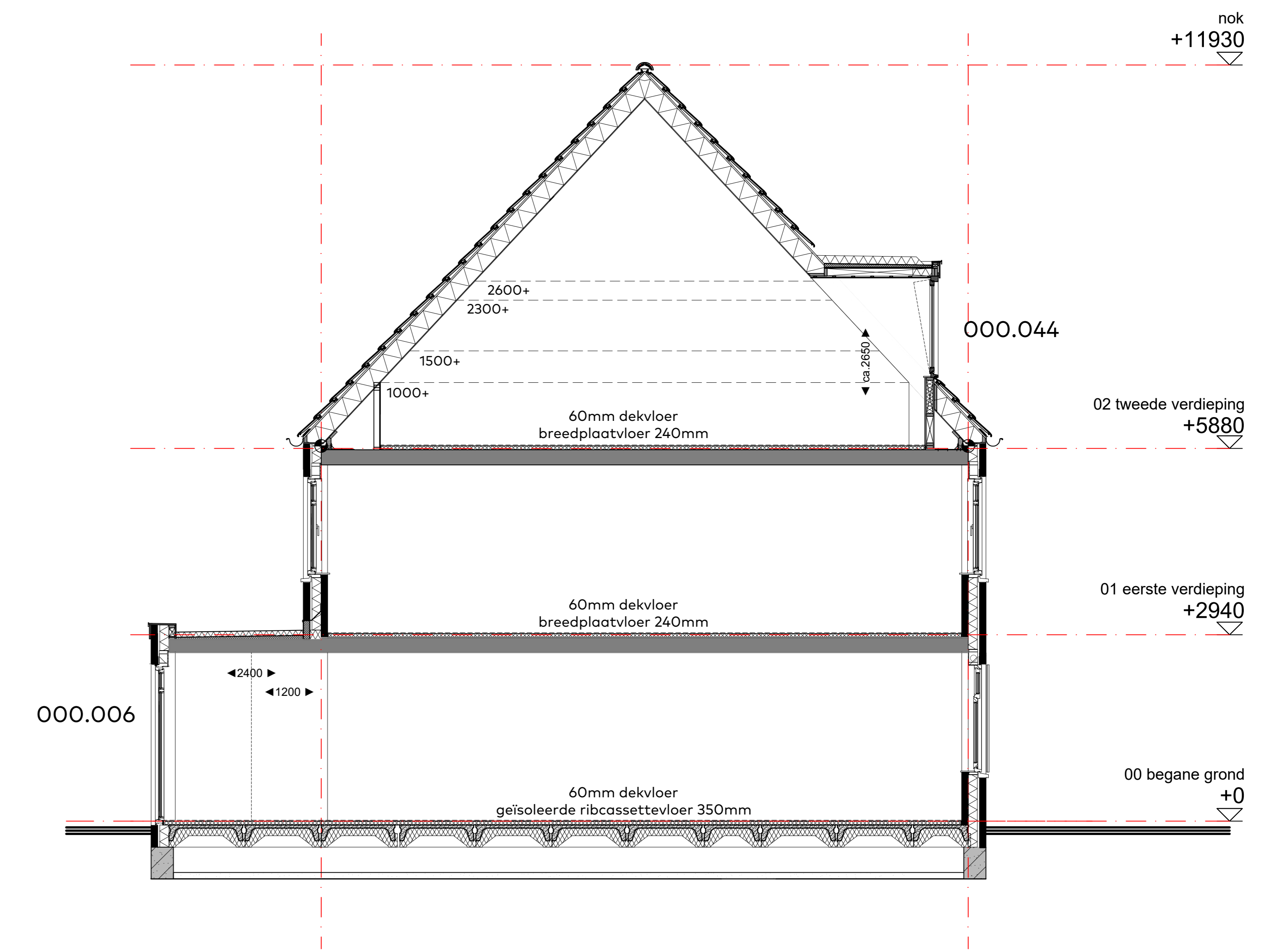
Doorsnede, blok E en F
